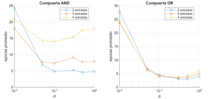
Figura 2. Épocas promedio hasta convergencia del perceptrón con la regla 3 en función de \alpha para AND y OR de 2, 3 y 4 entradas, 20 semillas.
